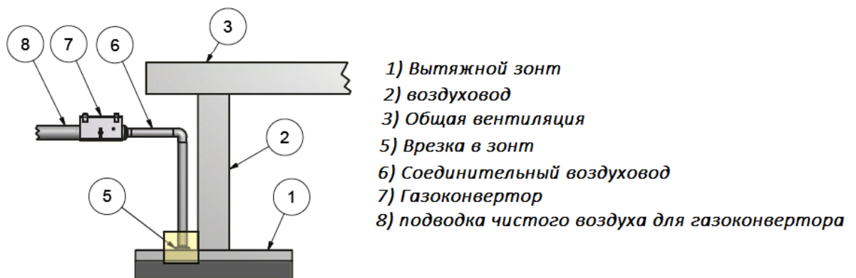
Рис. 6. Вариант подключения газоконвертора к вытяжному зонту.
