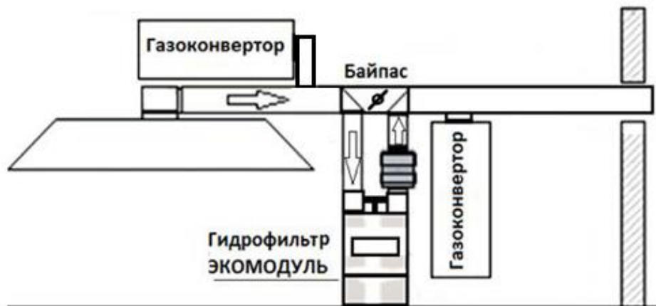
Рис. 4. Расположение газоконвертора «Экстра-Антизапах» в производственном помещении.
